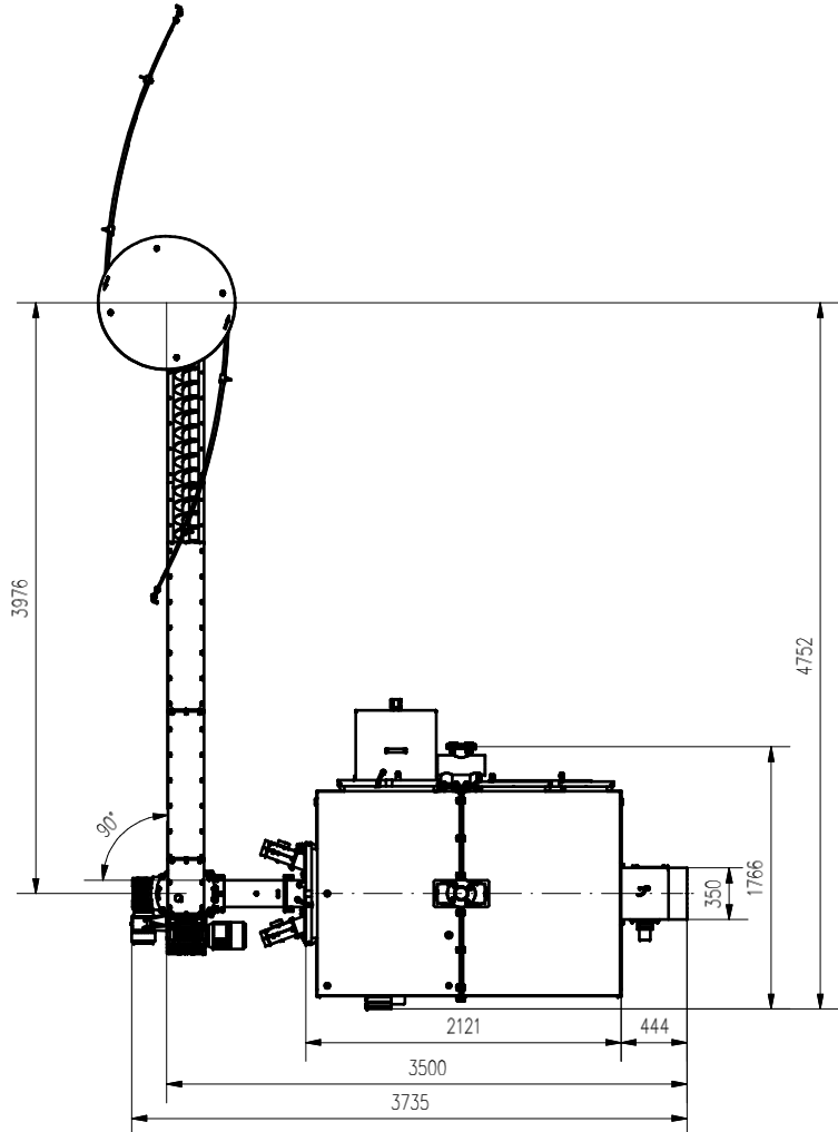
AZSB240GZ NS1604 F, L SUP P kat 90 L Maksymalny zakres pracy ramion sprężystych □3000 Podajnik można ustawić pod dowolnym kątem w stosunku do głowicy
